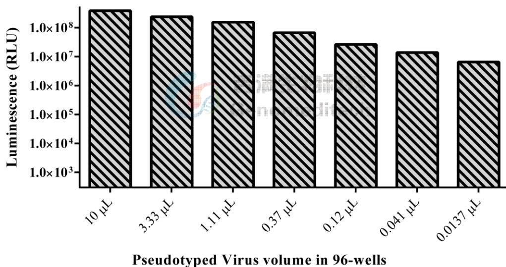
图2 吉满 SARS-CoV-2 Spike S 蛋白(XBB.1.6)突变型假病毒感染 HEK293T-ACE2 测定 Luciferase 数值
